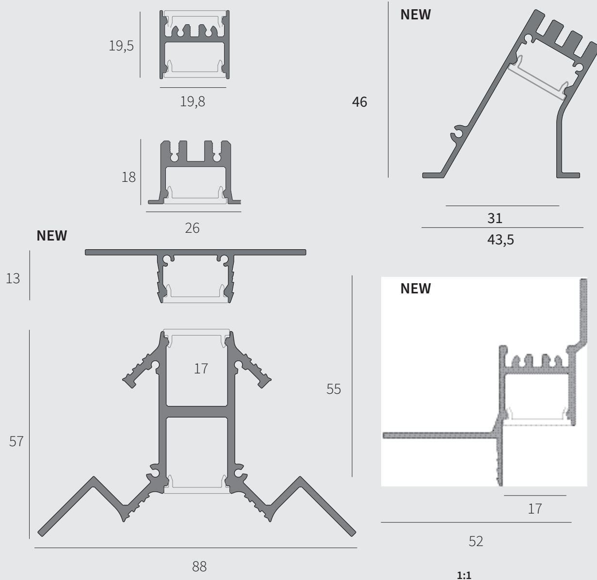
SEZIONE PROFILO/SECTION PROFILE
